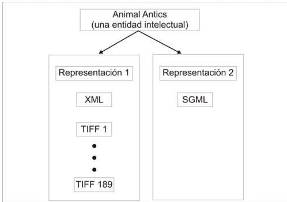
Gráfico 2: Ejemplo de la Entidad Intelectual Animal Antics
