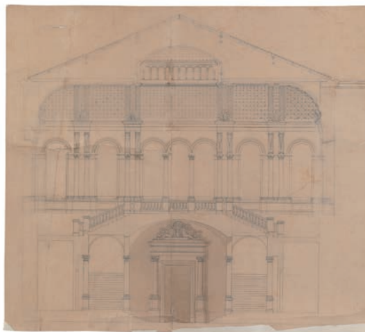
Sección del vestíbulo de la Biblioteca Nacional, A. Ruiz de Salces. BNE.
