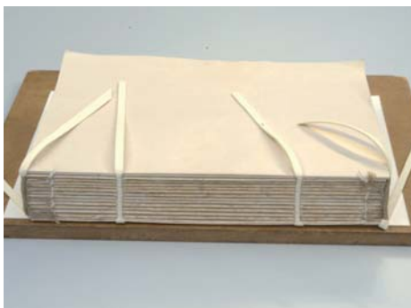
Estructura de cosido y cabezadas.
